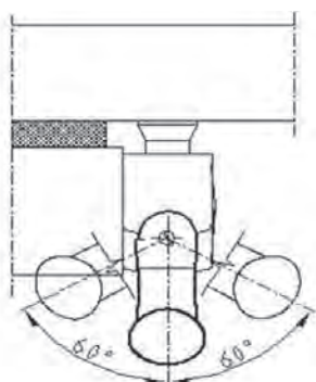
Possibili posizioni impugnatura Handle different positionings
