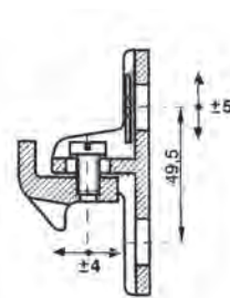
Aggancio regolabile Adjustable strike
